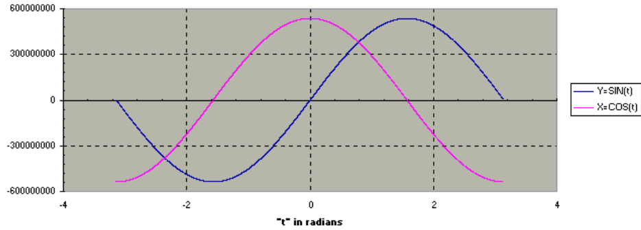
ATAN(Y, X)-Floating Point Computation (Q29)
