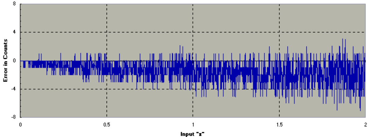
Error=IQ30sqrt(x)-SQRT(x)
